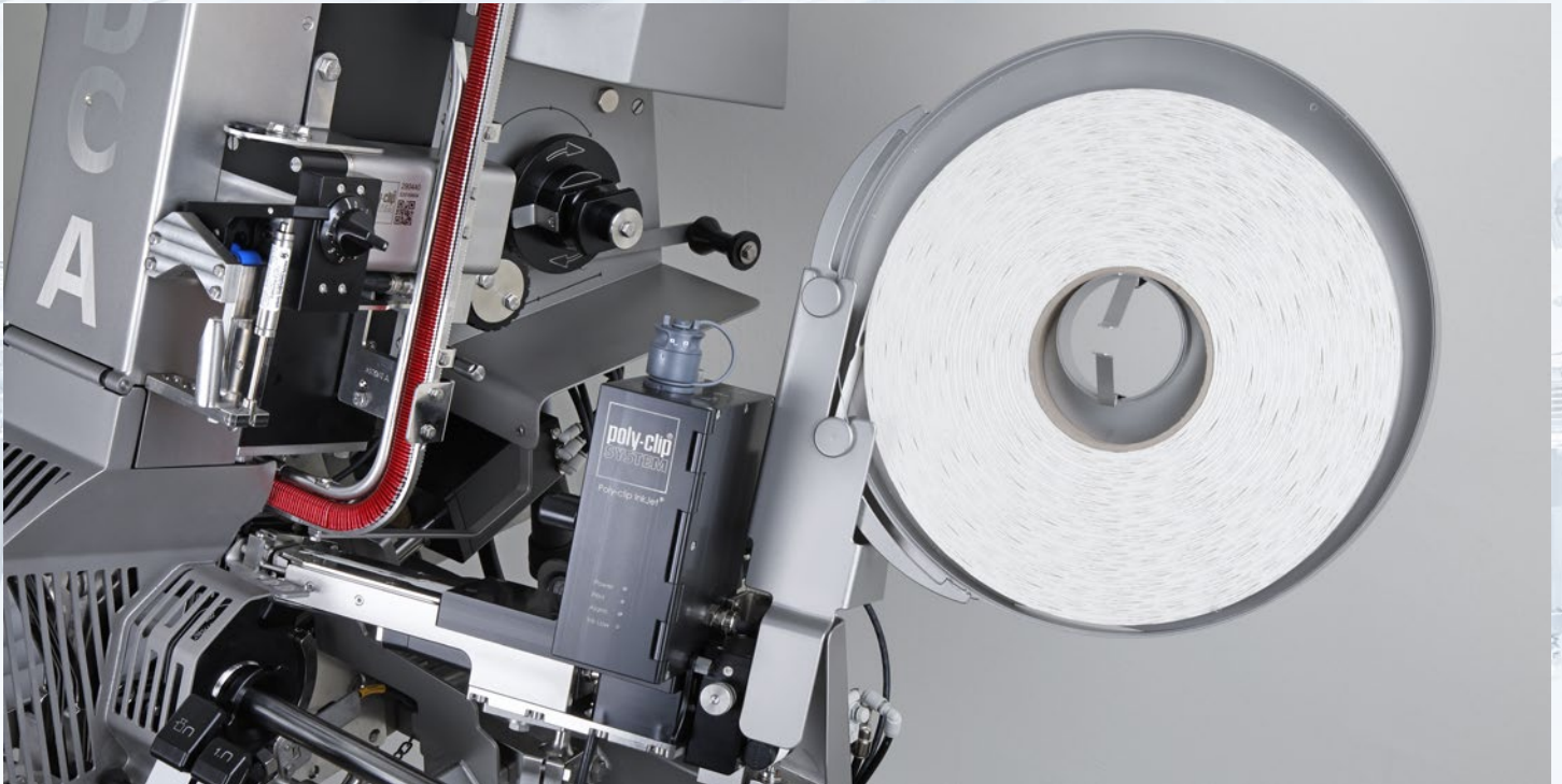
Gurtschlaufeneinleger GSE ist rechts an der Maschine befestigt.
