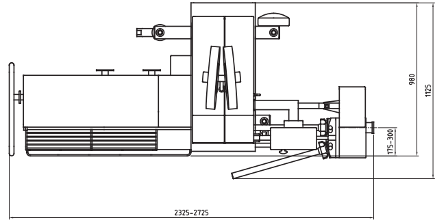
Draufsicht | Füllrohrlänge 600 (Abmessungen in mm)
