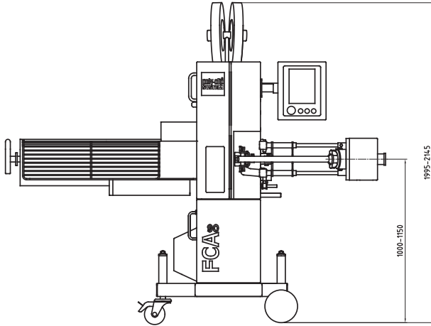
Vorderansicht (Abmessungen in mm)
